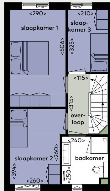
1e Verdieping
