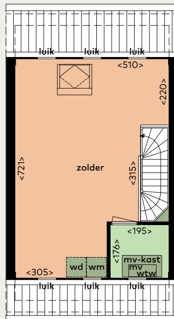
2e Verdieping
