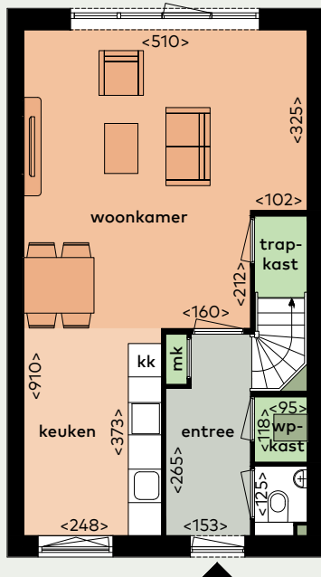
Begane Grond
