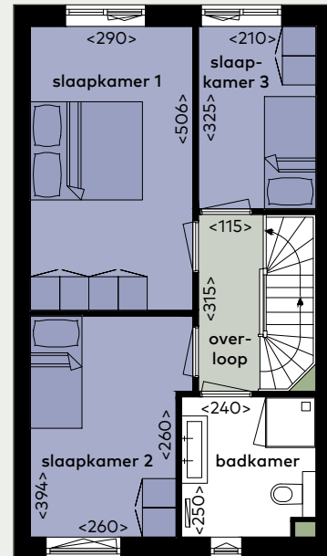
1e Verdieping
