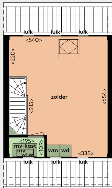
2e Verdieping
