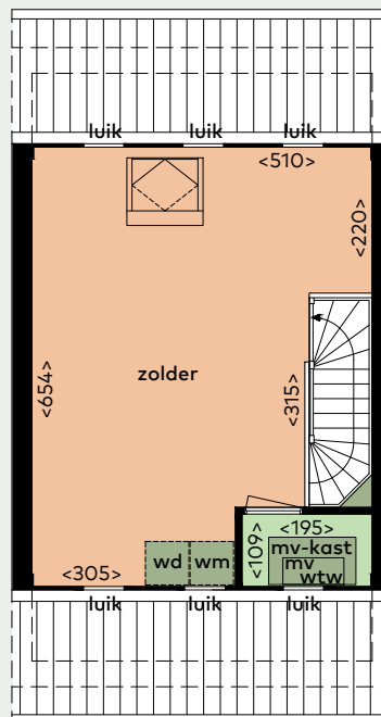
2e Verdieping
